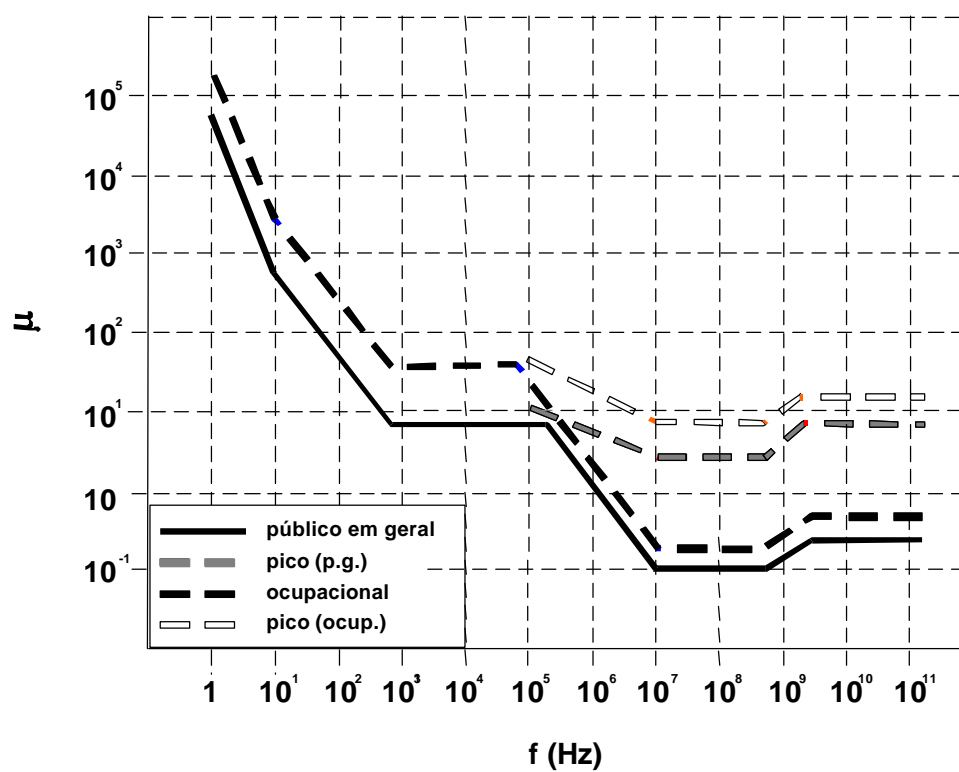
Fig. 2 – Níveis de referência para exposição a campos magnéticos variáveis no tempo (ver Tabelas 6 e 7).
