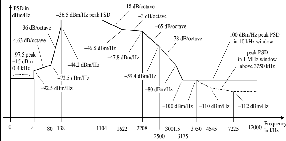
Figura 6 – Máscara de DEP para modems de central ADSL 2+ com espectro não sobreposto
