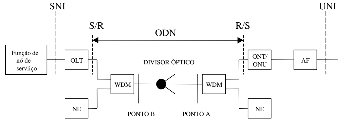
Figura 1 – Configuração da rede GPON
