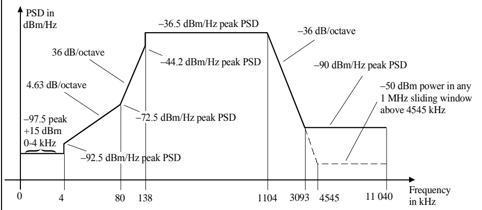
Figura 3 – Máscara da DEP para modems de central ADSL2 com espectro não sobreposto
