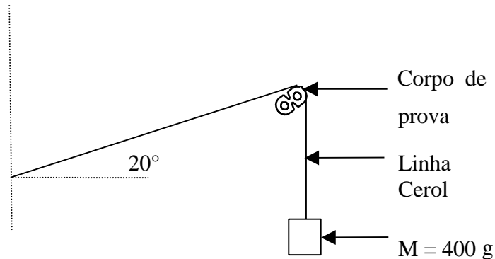
Figura 1 – Esquema do dispositivo para ensaio de resistência ao corte por linha cerol
