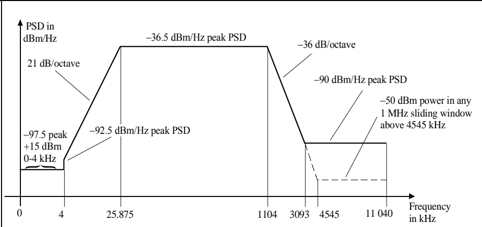
Figura 2 – Máscara de DEP para modems de central ADSL2 com espectro sobreposto
